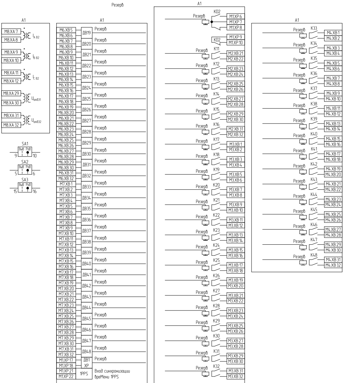
Рисунок В.3 – Схема электрическая принципиальная (часть 3)
